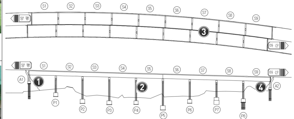
② 마산방향 P4 교평부 박락, 철근노출
