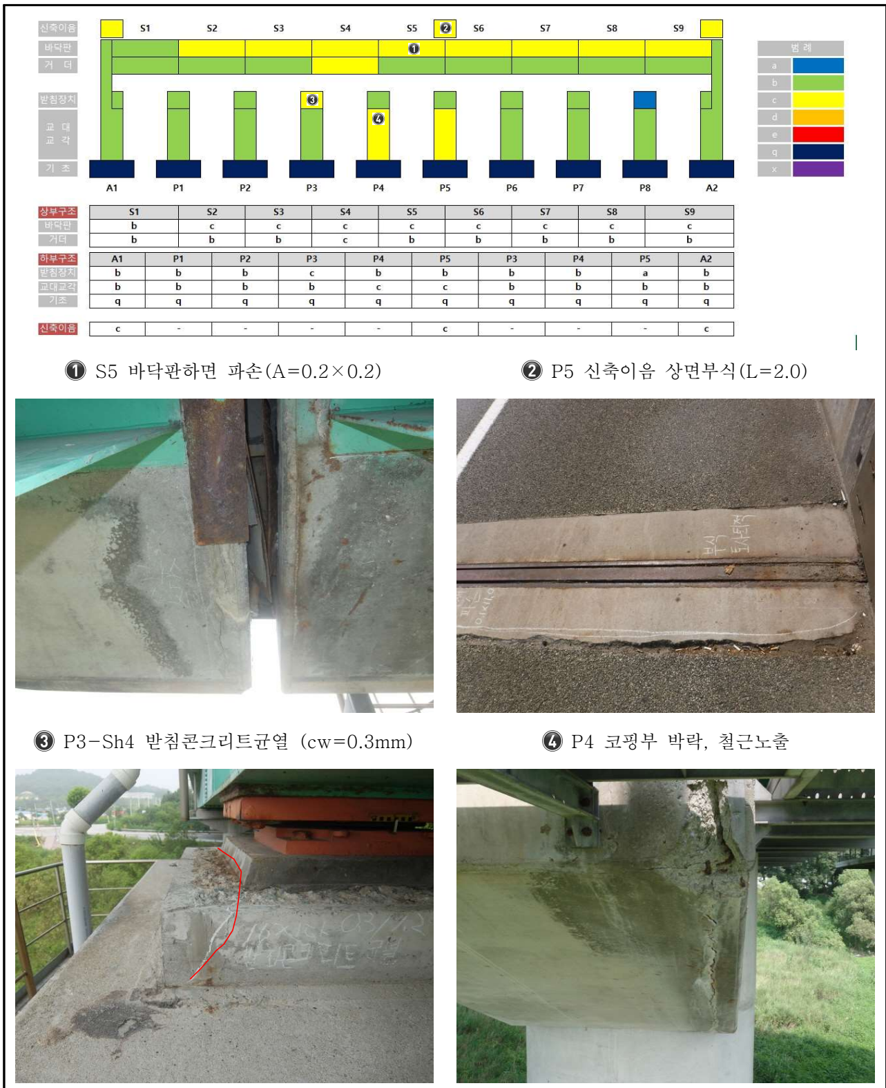
【그림 7-8】 마산방향 상태평가 현황도 및 주요 손상 위치도
