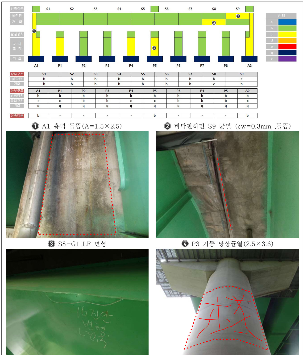
【그림 7-7】 양평방향 상태평가 현황도 및 주요 손상 위치도
