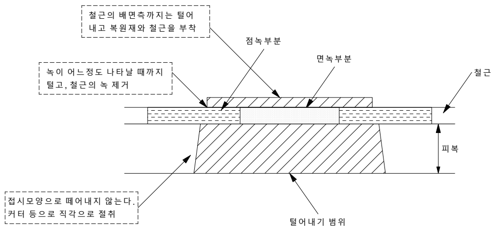
【그림 7-4】 단면복구 상세도
