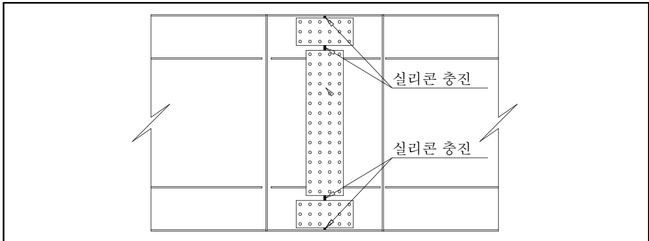
【그림 7-6】 스플라이스 틈새 실런트 주입
