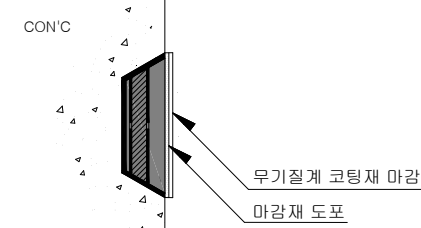
【그림 7-5】 단면복구(염해방지) 상세도
